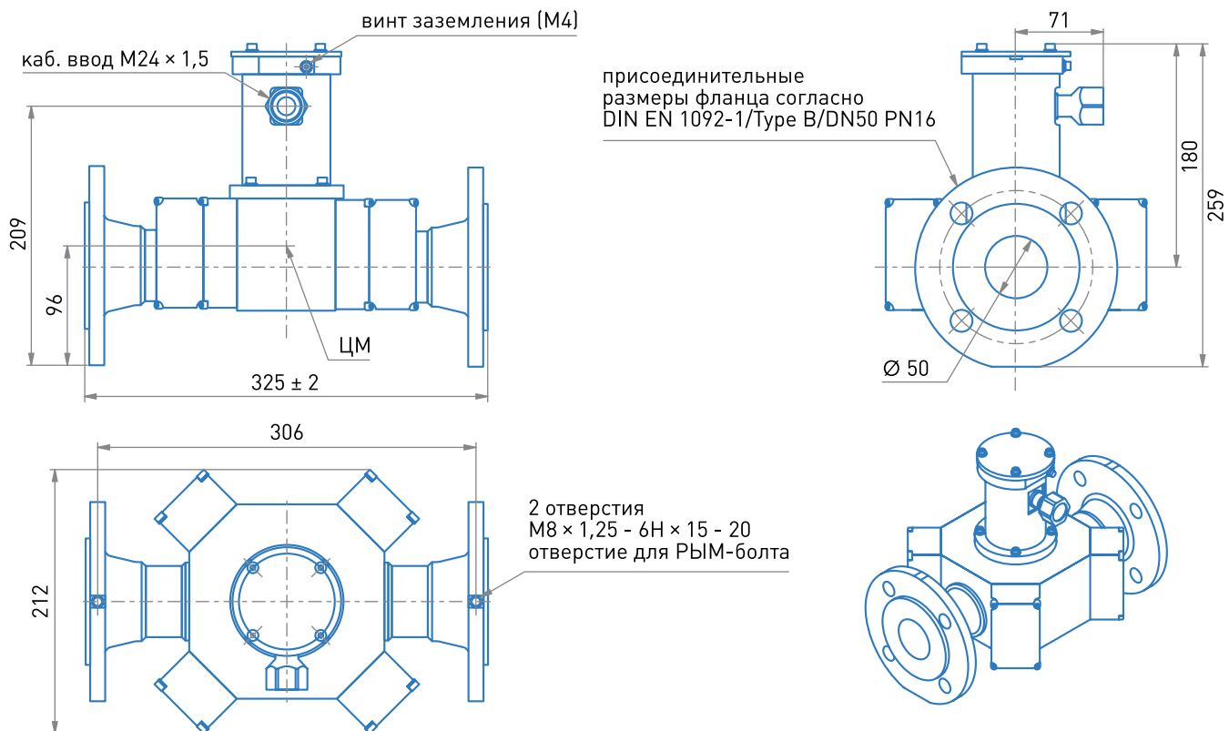
Габаритный чертеж расходомера ДУ 50
